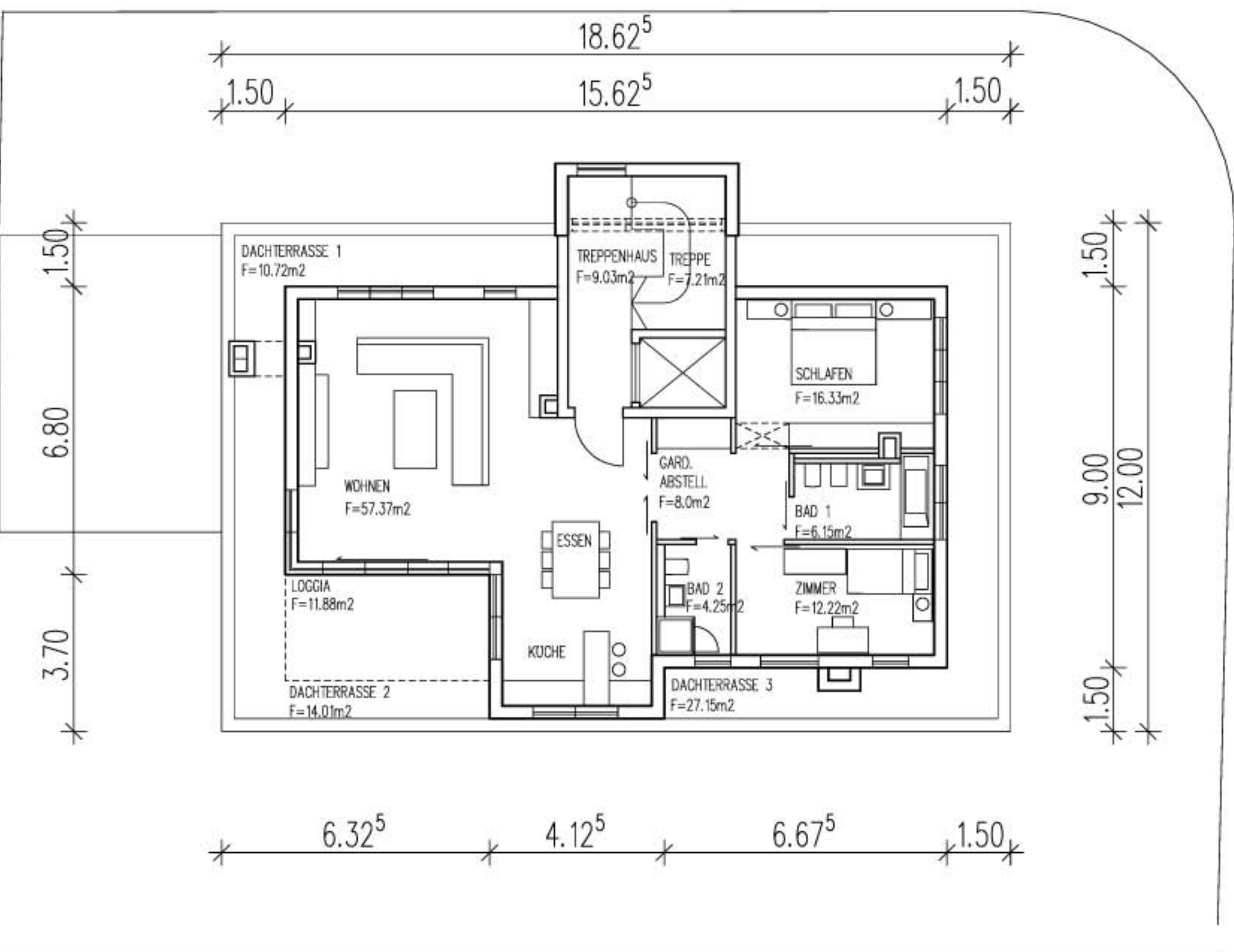
Grundriss DG
